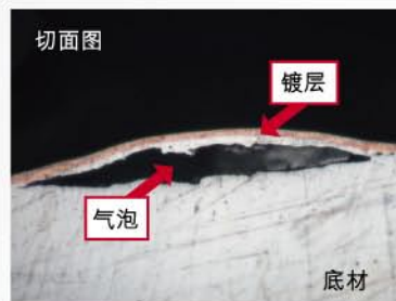
图2.3 起泡位置的横切面，冷纹造成起泡
