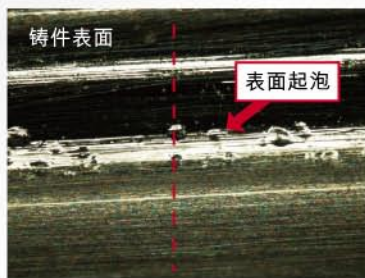
图2.2 沿红色虚线切开样本作金相分析
