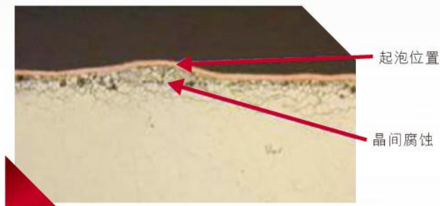
图二：金属基体表面出现明显晶间腐蚀
